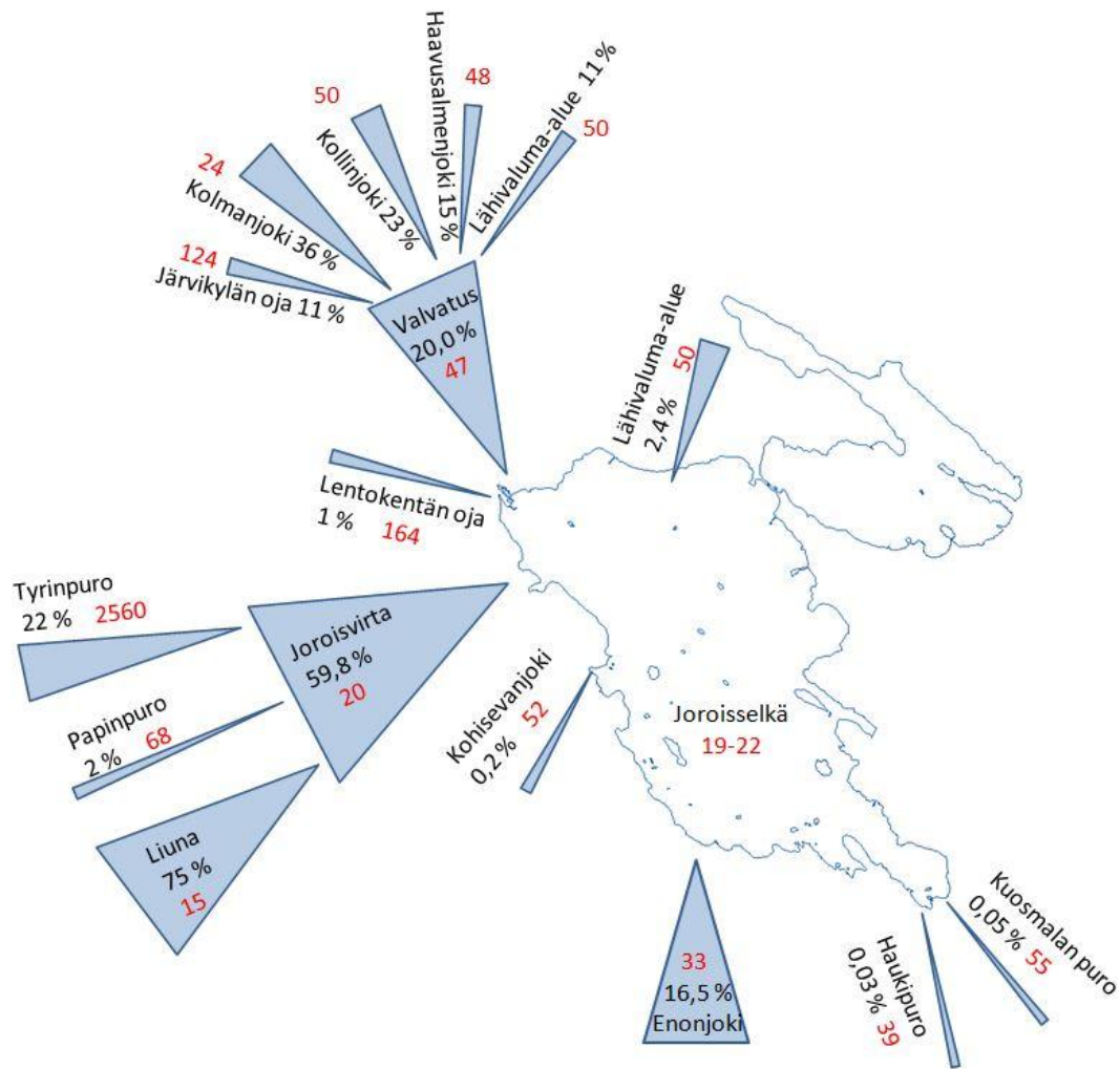
Kuva 9. Vesinäytteenottojen perusteella lasketut keskimääräiset ulkoisen fosforikuormituksen suhteelliset osuudet eri valuma-alueilta Joroisjärveen. Punaisella fontilla ovat keskimääräiset fosforipitoisuudet. Joroisjärven keskimääräinen fosforipitoisuus on pintaveden tuloksista 2000-luvulta.
