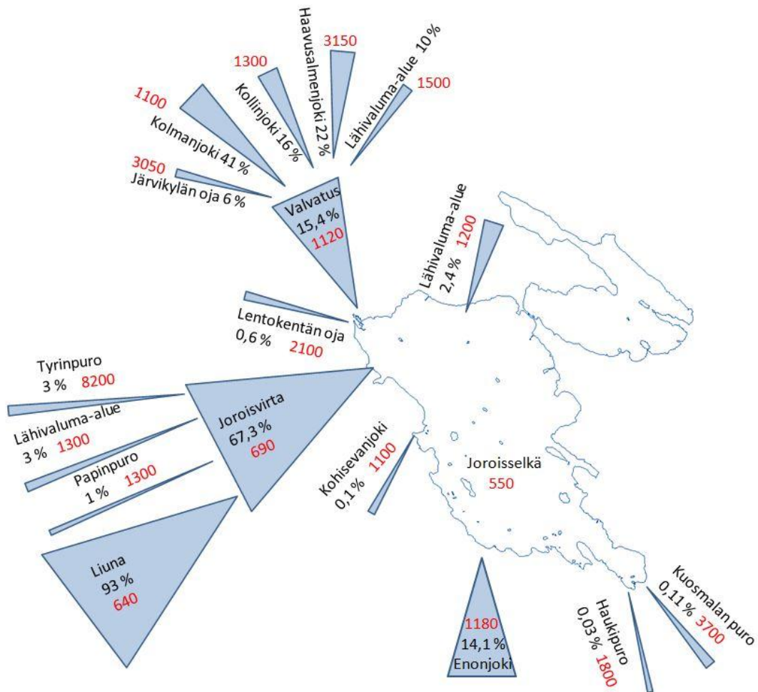
Kuva 10. Vesinäyteenottojen perusteella lasketut keskimääräiset ulkoisen typpikuormituksen suhteelliset osuudet eri valuma-alueilta Joroisellä. Punaisella fontilla ovat keskimääräiset typpipitoisuudet. Joroisellä keskimääräinen typpipitoisuus on pintaveden tulokista 2000-luvulta.
