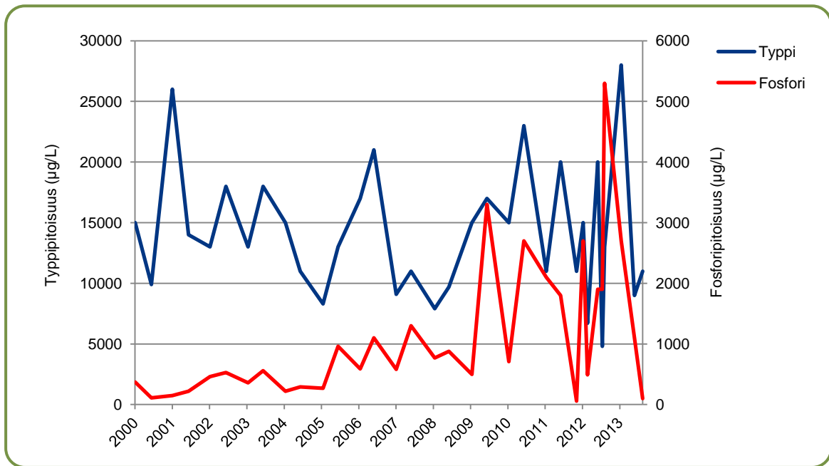
Kuva 5. Tyripuron vesinäytepisteeseen fosfori- ja typpipitoisuudet 2000-luvulla.
