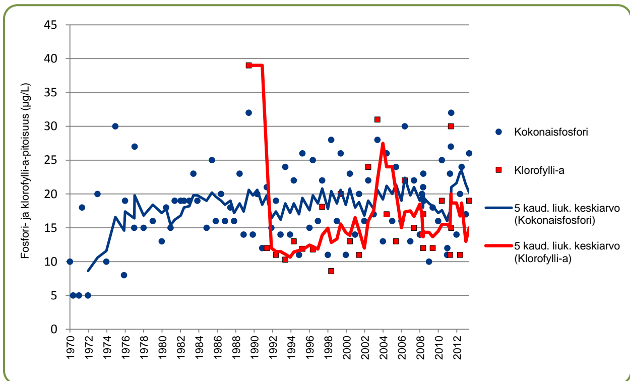
Kuva 2. Joroisselän kokonaisfosfori- ja klorofylli-a-pitoisuudet seuratuimmasta vedenlaatu pisteestä (Joroisselkä 012). Kokonaisfosforipitoisuudet ovat pintaveden tuloksia ja klorofylli-a:n tulokset kokoomanäytteen tuloksia (0-2 m veden pinnasta).
